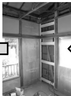
補強壁設置中
